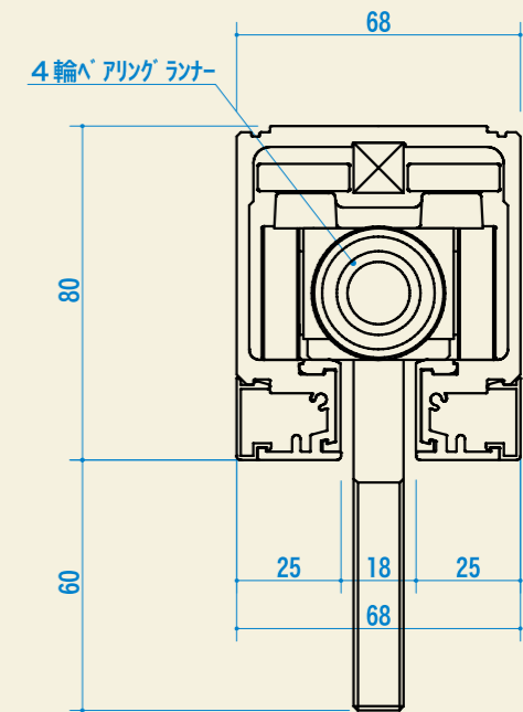
型材断面詳細図
